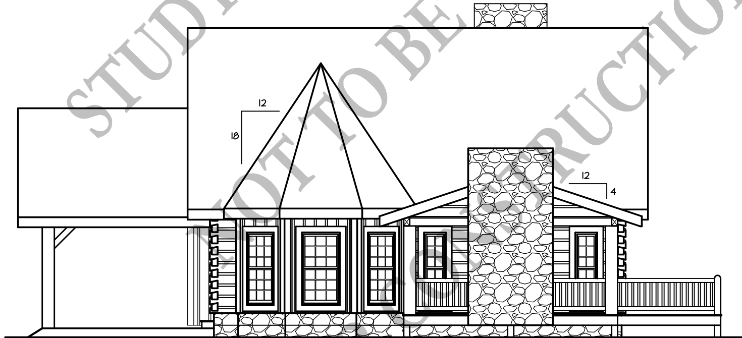
RIGHT ELEVATION
